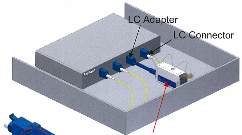
One-Click Cleaner MU/LC Mini
